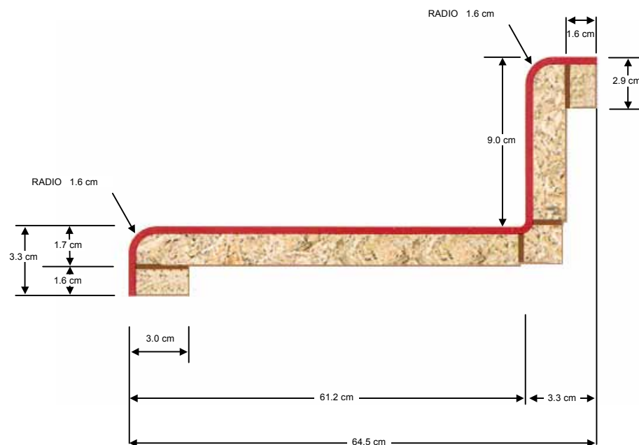
CUBIERTA MODELO ESTÁNDAR MEDIDAS DISPONIBLES (2.40, 3.00 Y 3.60)
