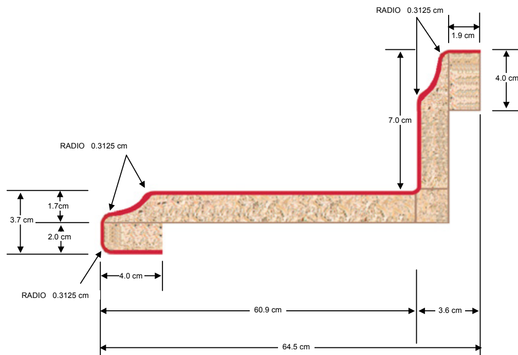
CUBIERTA MODELO CASCADA MEDIDAS DISPONIBLES (2.40, 3.00 Y 3.60)
