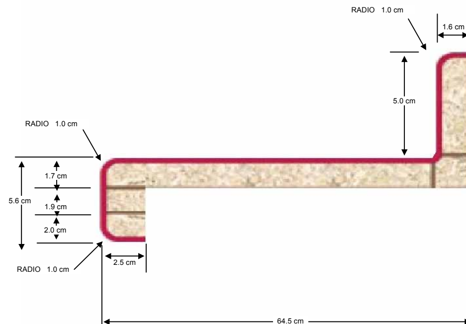
CUBIERTA MODELO CUADRADA 2-E19 MEDIDAS DISPONIBLES (2.40, 3.00 Y 3.60)
